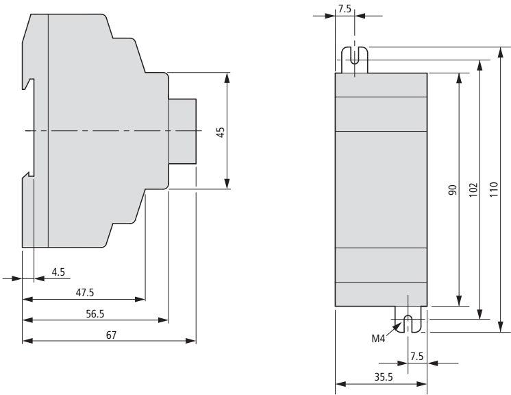
Abbildung 26: Abmessung EASY221-CO, Maße in mm
