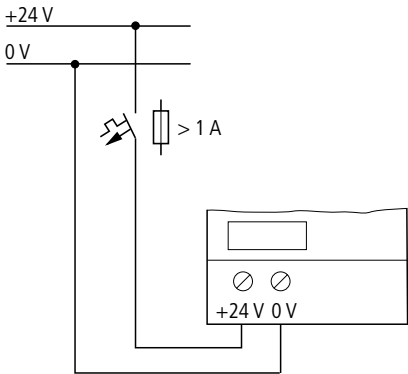
Abbildung 5: Versorgungsspannung EASY221-CO
