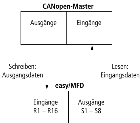
Abbildung 25: Ein- und Ausgangsdaten aus Sicht des CANopen-Masters
