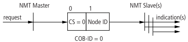
Abbildung 13: Aufbau der NMT Services, Start Remote Node
