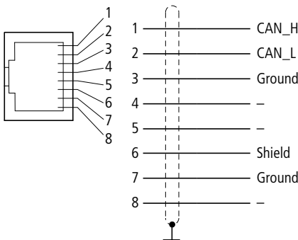
Abbildung 6: Anschlussbelegung Gerätebuchse
