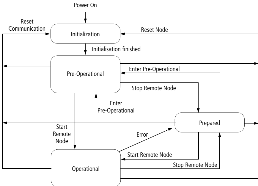
Abbildung 12: Netzwerkmanagement
