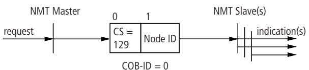
Abbildung 16: Aufbau der NMT Services, Reset Node
