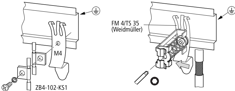
Abbildung 8: Schirmbefestigung auf Hutschiene
