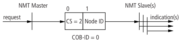
Abbildung 14: Aufbau der NMT Services, Stop Remote Node
