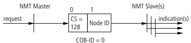
Abbildung 15: Aufbau der NMT Services, Pre Operational State
