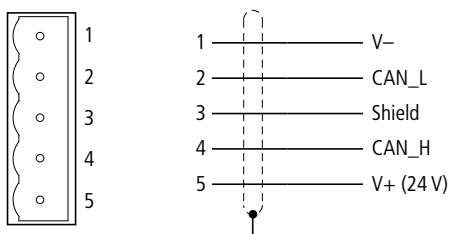
Abbildung 6: Anschlussbelegung Gerätebuchse
