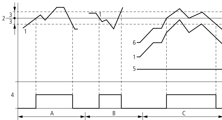
Figura 72: Diagramma di stato "Comparatore valori analogici"
