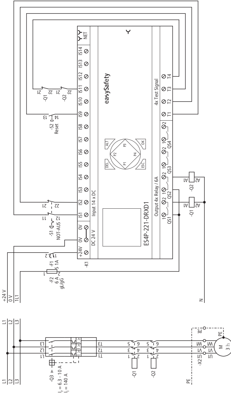
Figura 175: Esempio "Ritorno": schema elettrico
