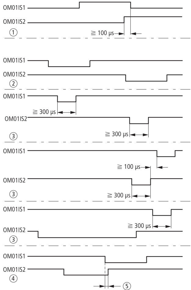
Figura 227: Andamento temporale dei segnali su IS1/IS2
