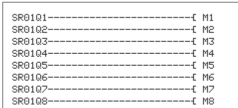
Figura 144: Modalità BIT, Cablaggio dei contatti del modulo
