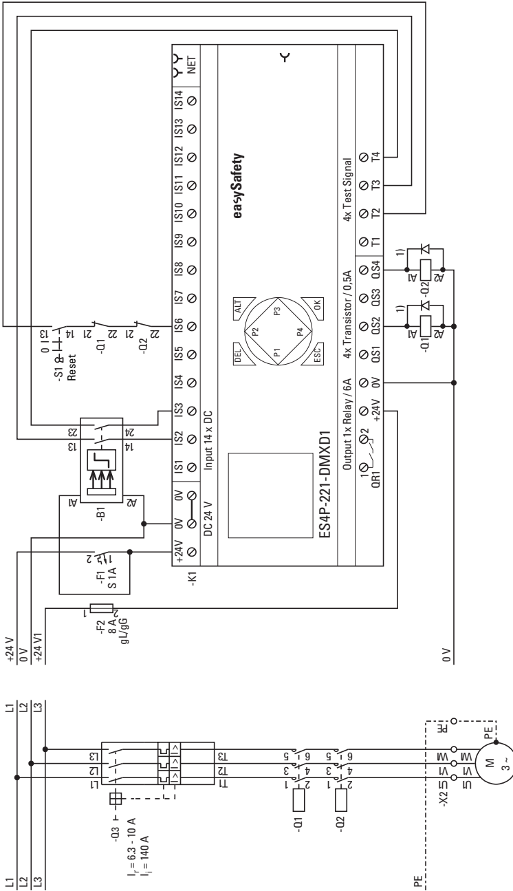
Figura 205: Esempio 2 "Griglia ottica"; schema elettrico 1) Utilizzare diodi soppressori per apparecchi ES4P-221-DMX... di versione 02 e 10
