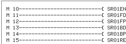
Figura 143: Modalità BIT, cablaggio delle bobine del modulo
