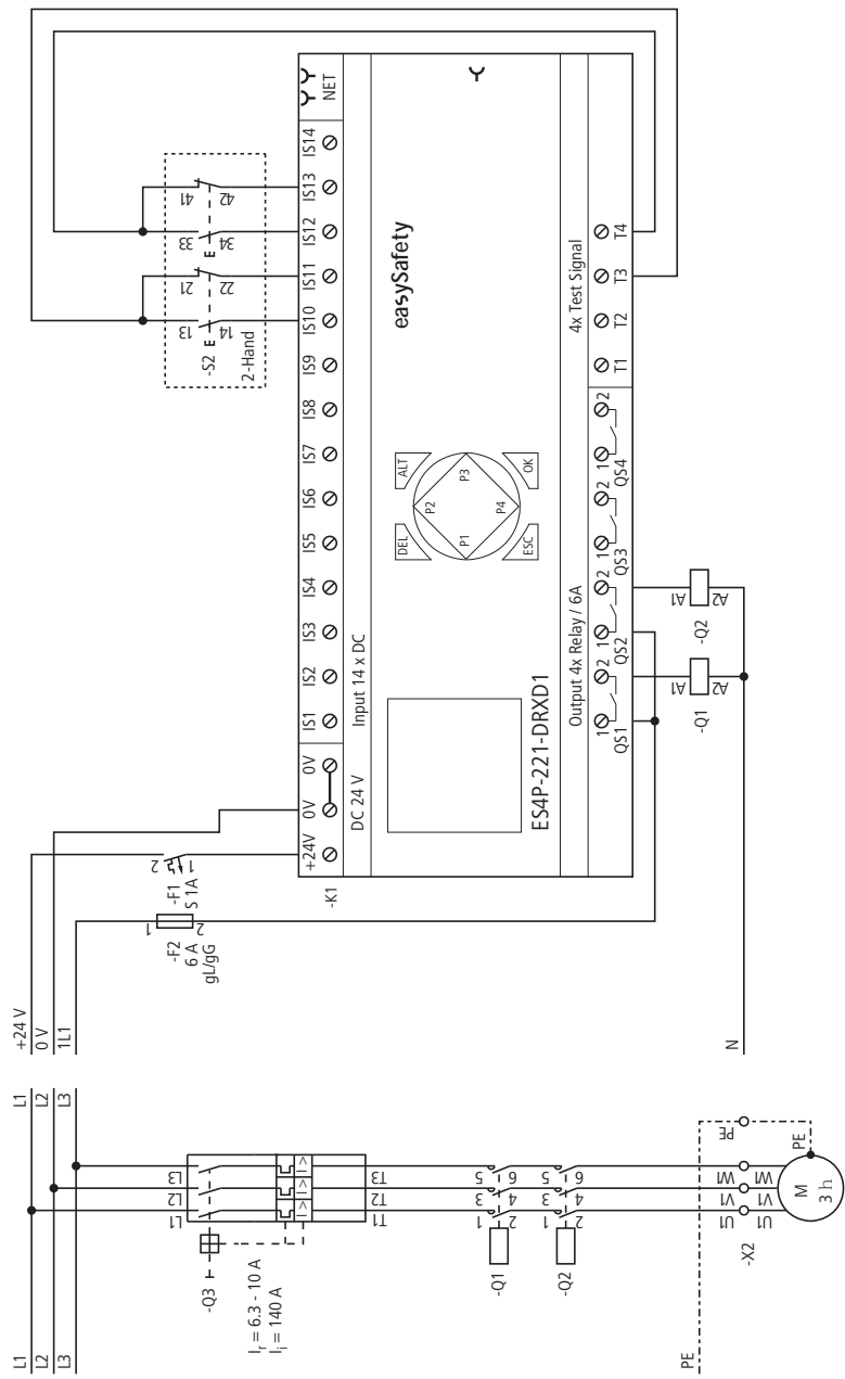
Figura 254: Esempio 2 "Tasto a due mani": schema elettrico
