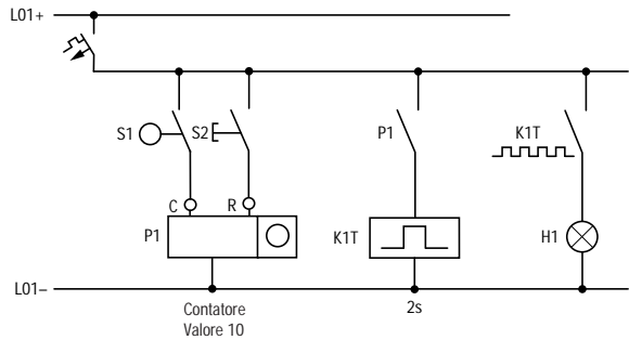
Figura 169: Cablaggio fisso con relè
