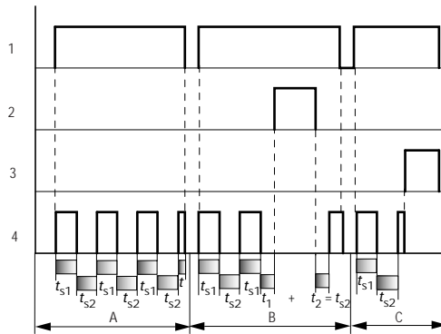
Figura 164: Diagramma di stato "Temporizzatore", lampeggiante in modo sincrono e asincrono
