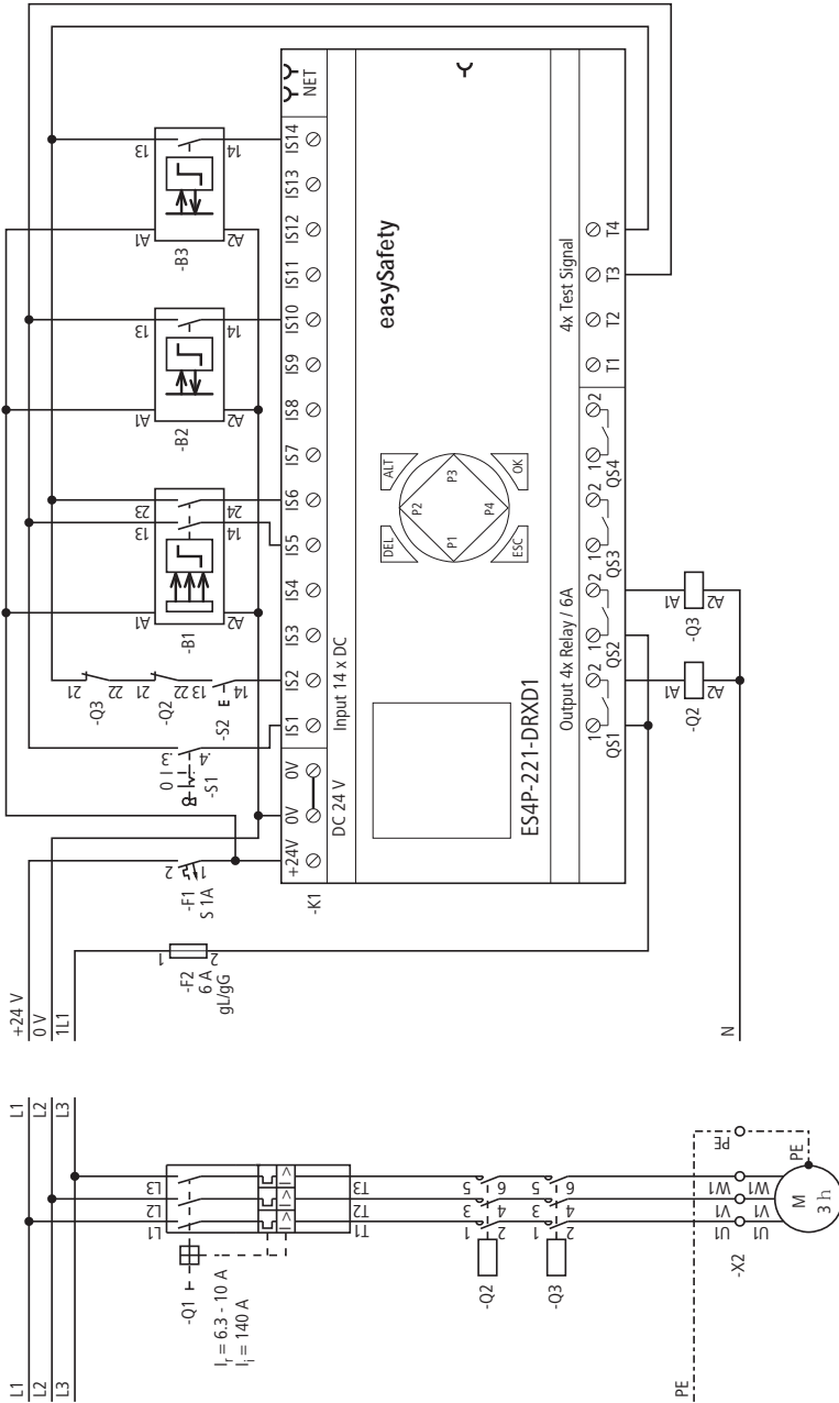
Figura 217: Esempio "Muting griglia ottica": schema elettrico
