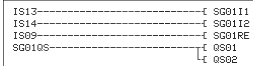
Figura 243: Esempio 1 "Porta di sicurezza": schema elettrico in easySafety
