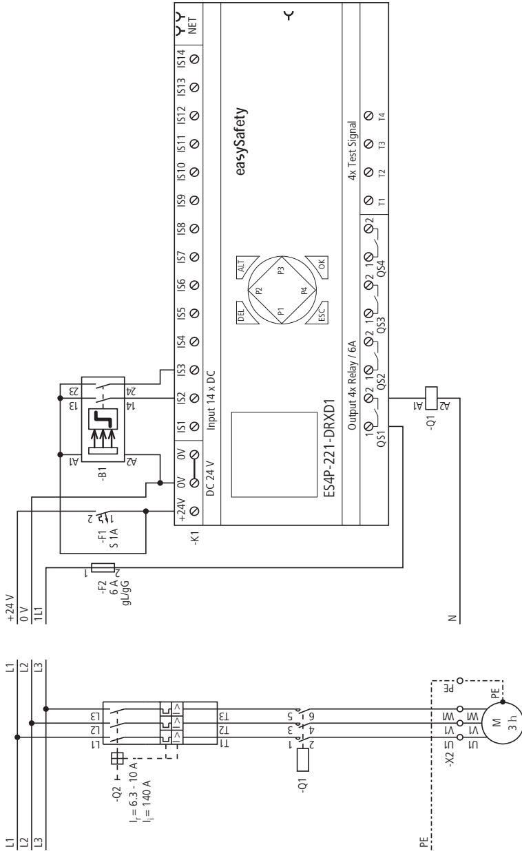
Figura 202: Esempio 1 "Griglia ottica" : schema elettrico
