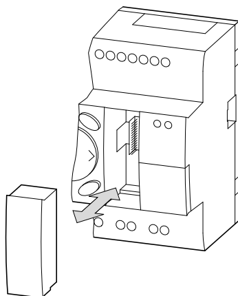
Figura 26: Inserire/rimuovere la copertura dell'interfaccia
