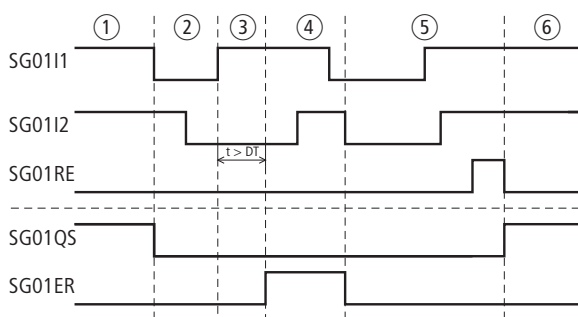
Figura 244: Esempio 1 "Porta di sicurezza": diagramma temporale
