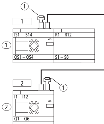
Figura 278: Esempio di topologia con due utenti NET
