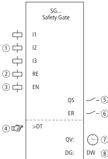
Figura 239: Modulo funzionale "porta di sicurezza"
