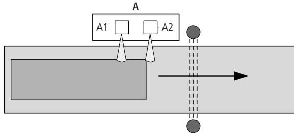
Figura 214: Muting griglia ottica: muting sequenziale con 2 sensori muting
