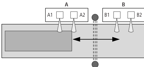
Figura 215: Muting griglia ottica: muting sequenziale con 4 sensori muting
