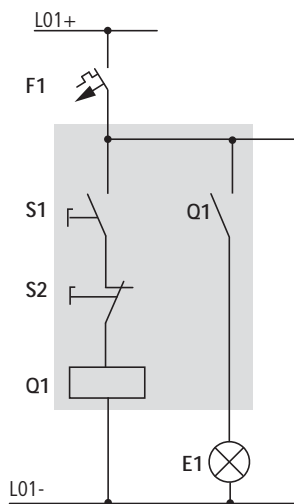
Figura 33: Comando di lampade tramite relè
