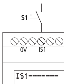
Figura 292: Ingresso easySafety configurato con interruttore
