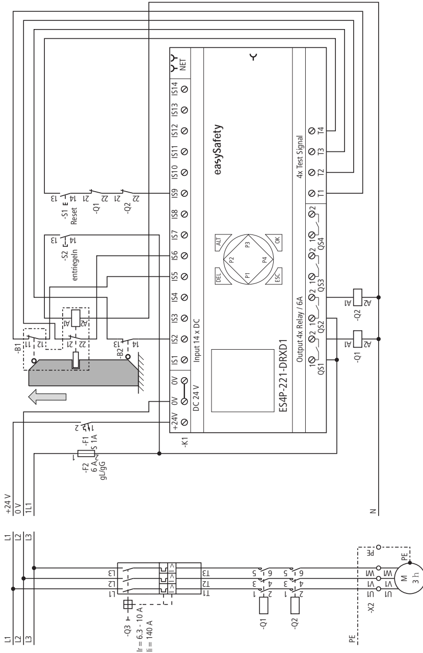
Figura 245: Esempio 2 "Porta di sicurezza": schema elettrico
