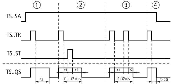
Figura 261: Diagramma d'azione "Temporizzatore ritardato alla diseccitazione"
