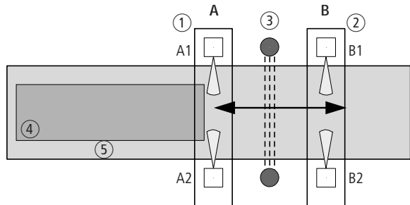
Figura 211: Muting griglia ottica: figura d'esempio, la direzione della freccia indica la possibile direzione del movimento del bene trasportato supportata dal procedimento di muting.
