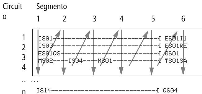
Schema elettrico standard
