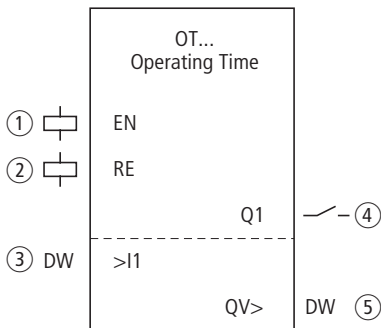
Figura 132: Modulo funzionale "Contaore"
