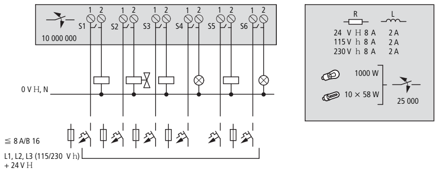
Figura 16: Uscite a relè EASY6...-RE..
