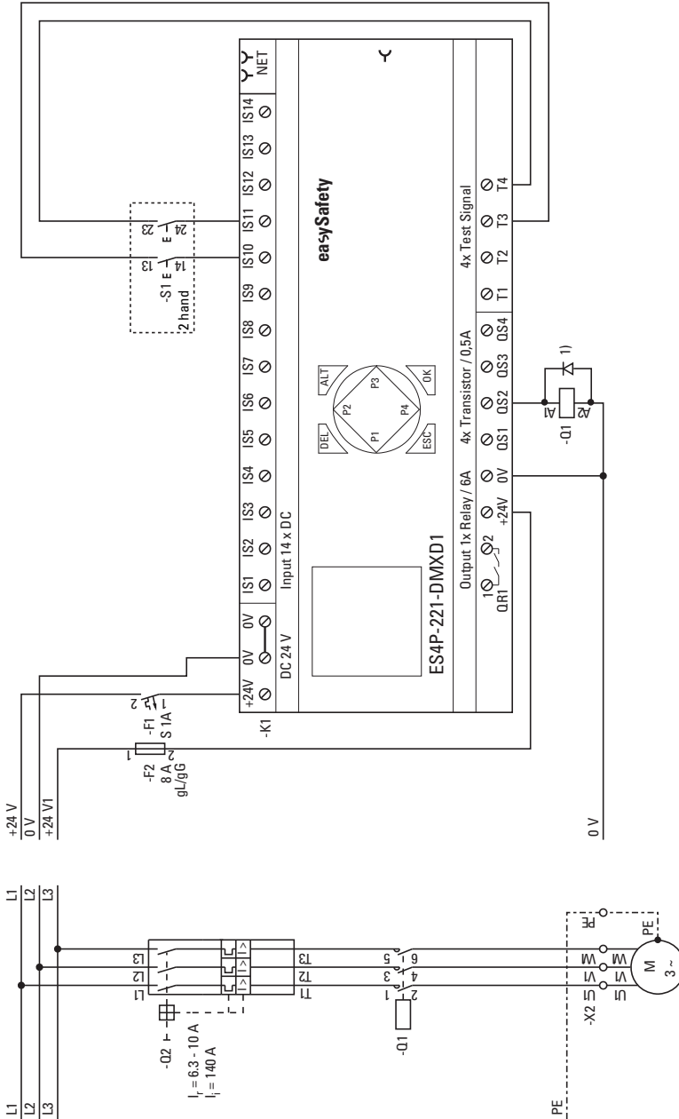
Figura 251: Esempio 1 "Tasto a due mani": schema elettrico 1) Utilizzare diodi soppressori per apparecchi ES4P-221-DMX.. di versione 02 e 10
