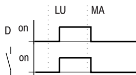
Figura 107: Diagramma di stato "Inserzione notturna"
