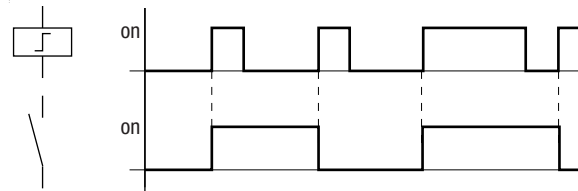
Abbildung 120:Wirkdiagramm „Stromstoßrelais“
