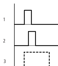
Abbildung 195:Wirkdiagramm PUT-Baustein
