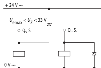
Abbildung 66: Induktivität mit Schutzbeschaltung
