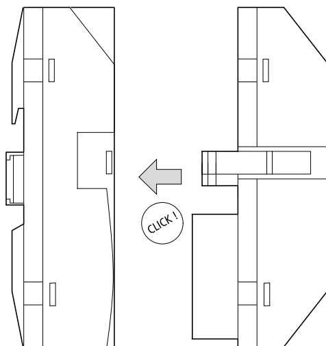
Abbildung 19: Ein-/Ausgangsmodule stecken
