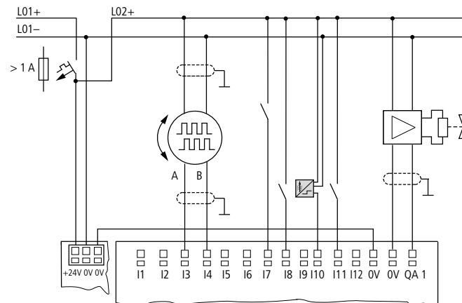
Abbildung 67: Servoventil anschließen
