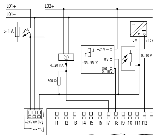
Abbildung 57: MFD-R.16(17) und MFD-T.16(17) mit Temperatur-, Helligkeits- und 20-mA-Sensor
