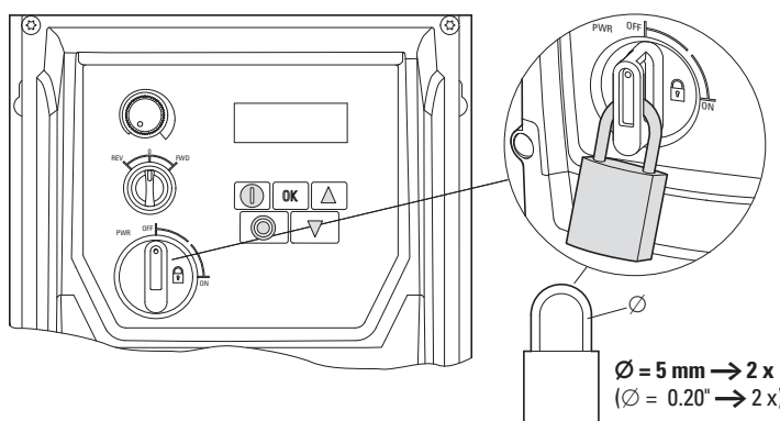
Ilustracja 33: DC1-...-A6SN z kłódką
