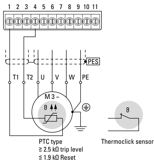
Ilustracja 60: Przyłącze termistora
