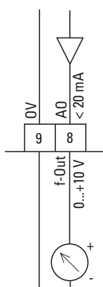
Ilustracja 56: Wyjście analogowe (AO) (przykład podłączenia)
