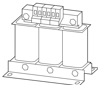
Ilustracja 81: Dławiki sieciowe DEX-LN3... (3-fazowe)
