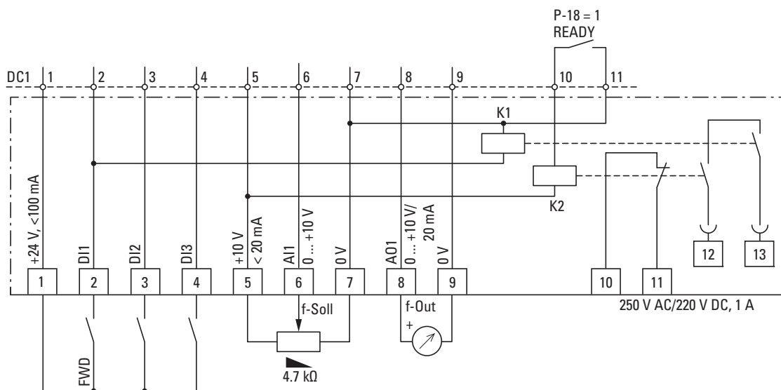
Ilustracja 92: Schemat blokowy DXC-EXT-2RO1AO
