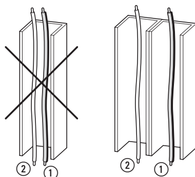
Ilustracja 35: Oddzielne układanie przewodów
