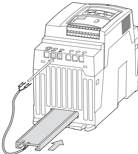
Ilustracja 15: Przekształtnik częstotliwości DC1 o wielkości FS2 z rezystorem hamowania DX-BR3-100
