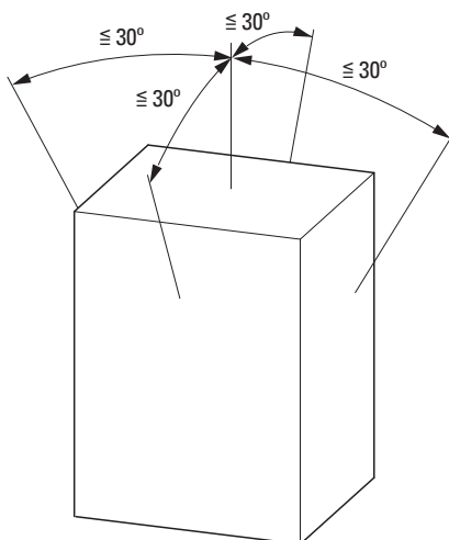
Ilustracja 23: Pozycja montażu
