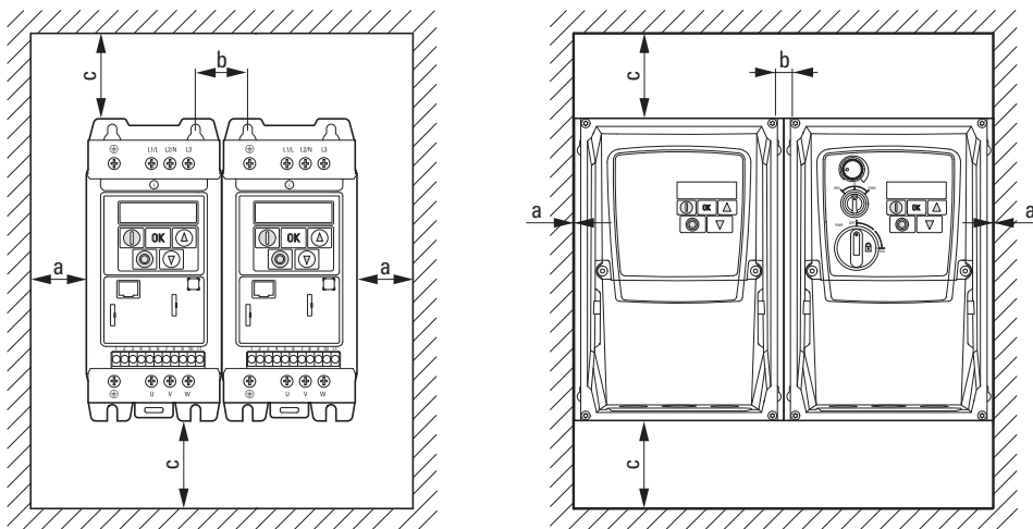
Figura 24: Spazi liberi per il raffreddamento ad aria (a sinistra IP20, a destra IP66)
