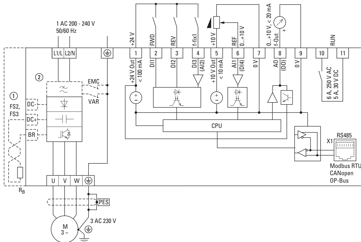
Figura 62: Schema a blocchi DC1-12...
