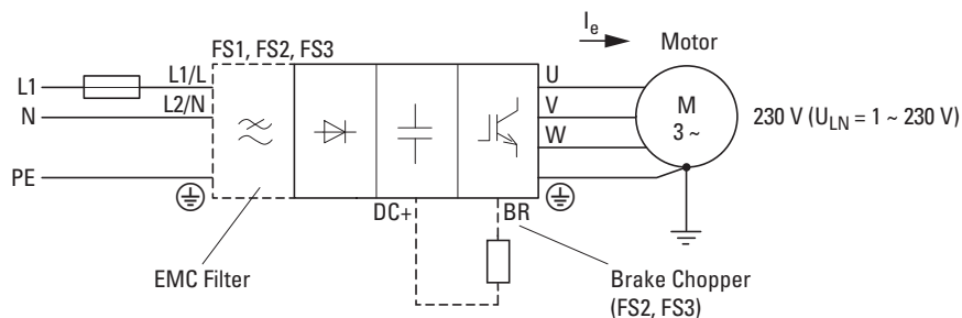
Figura 9: DC1-12...
