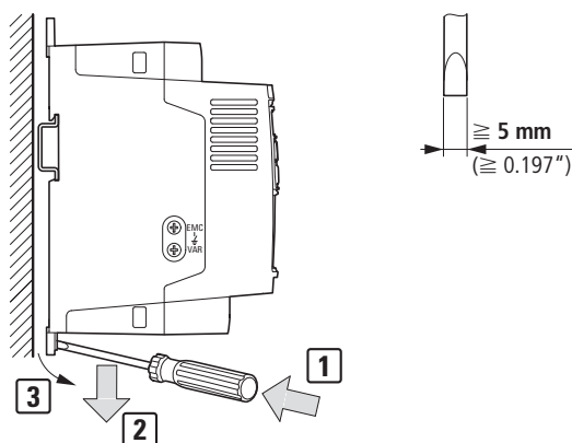
Figura 30: Smontaggio della guida di montaggio
