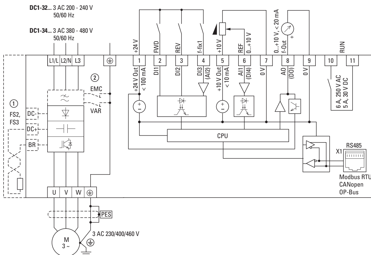
Figura 63: Schema a blocchi DC1-32... e DC1-34... nelle grandezze FS1, FS2 e FS3
