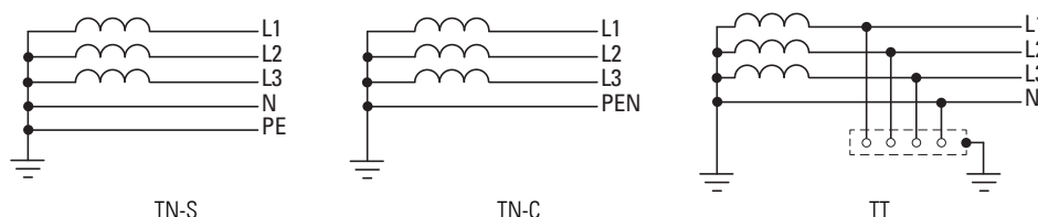
Figura 14: Reti a corrente alternata con punto centrale messo a terra
