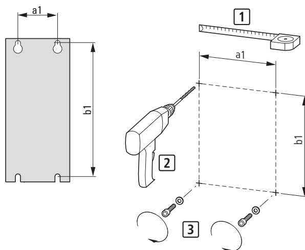
Figura 27: Quote di montaggio
