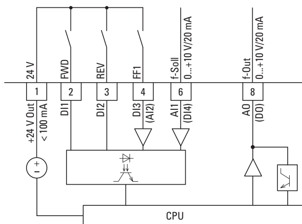
Figura 54: Morsetti di comando (D = digitali/A = analogici)
