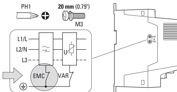
Figura 36: Vite EMC e VAR
