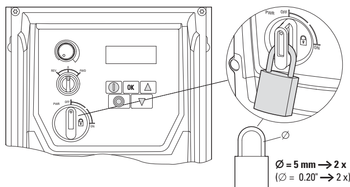
Figura 33: DC1-...-A6SN con lucchetto
