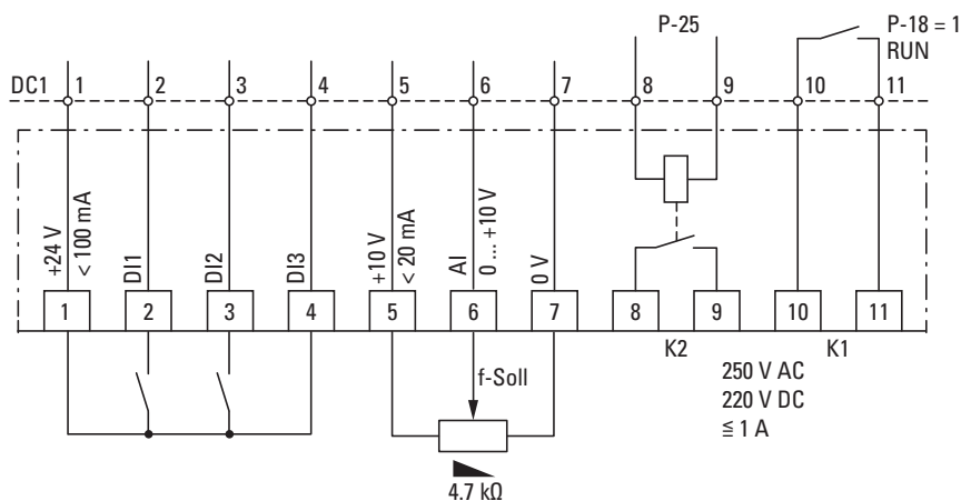
Figura 88: Schema a blocchi DXC-EXT-2RO
