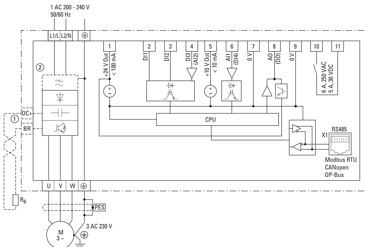
Figura 68: Schema a blocchi DC1-12...-A66...
