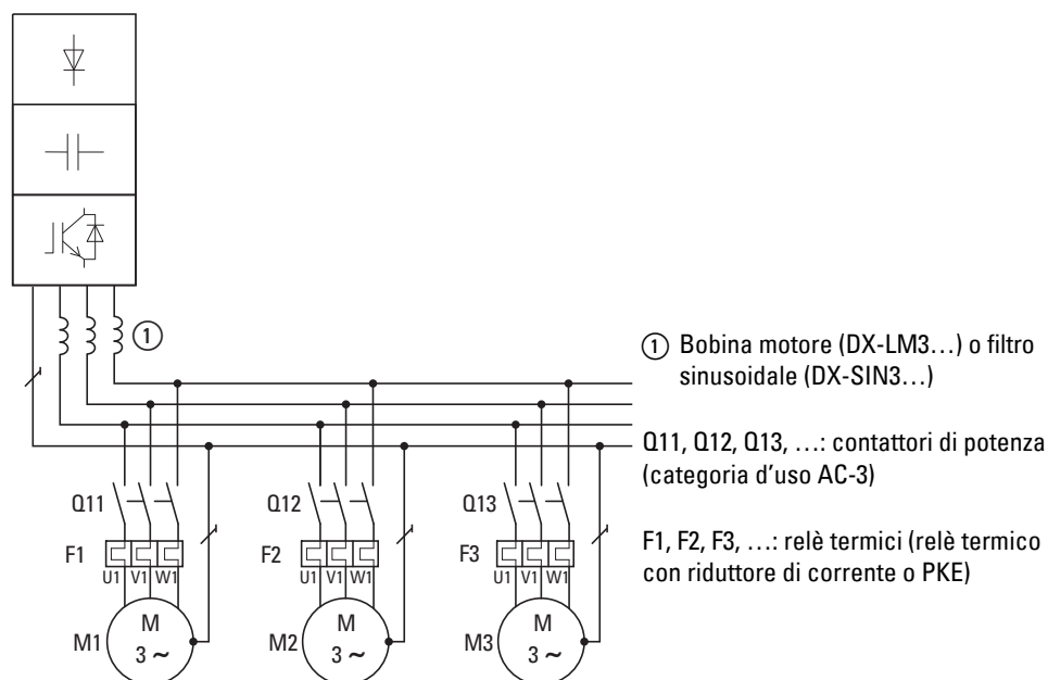
Figura 19: Esempio: Collegamento in parallelo di più motori sullo stesso convertitore di frequenza
