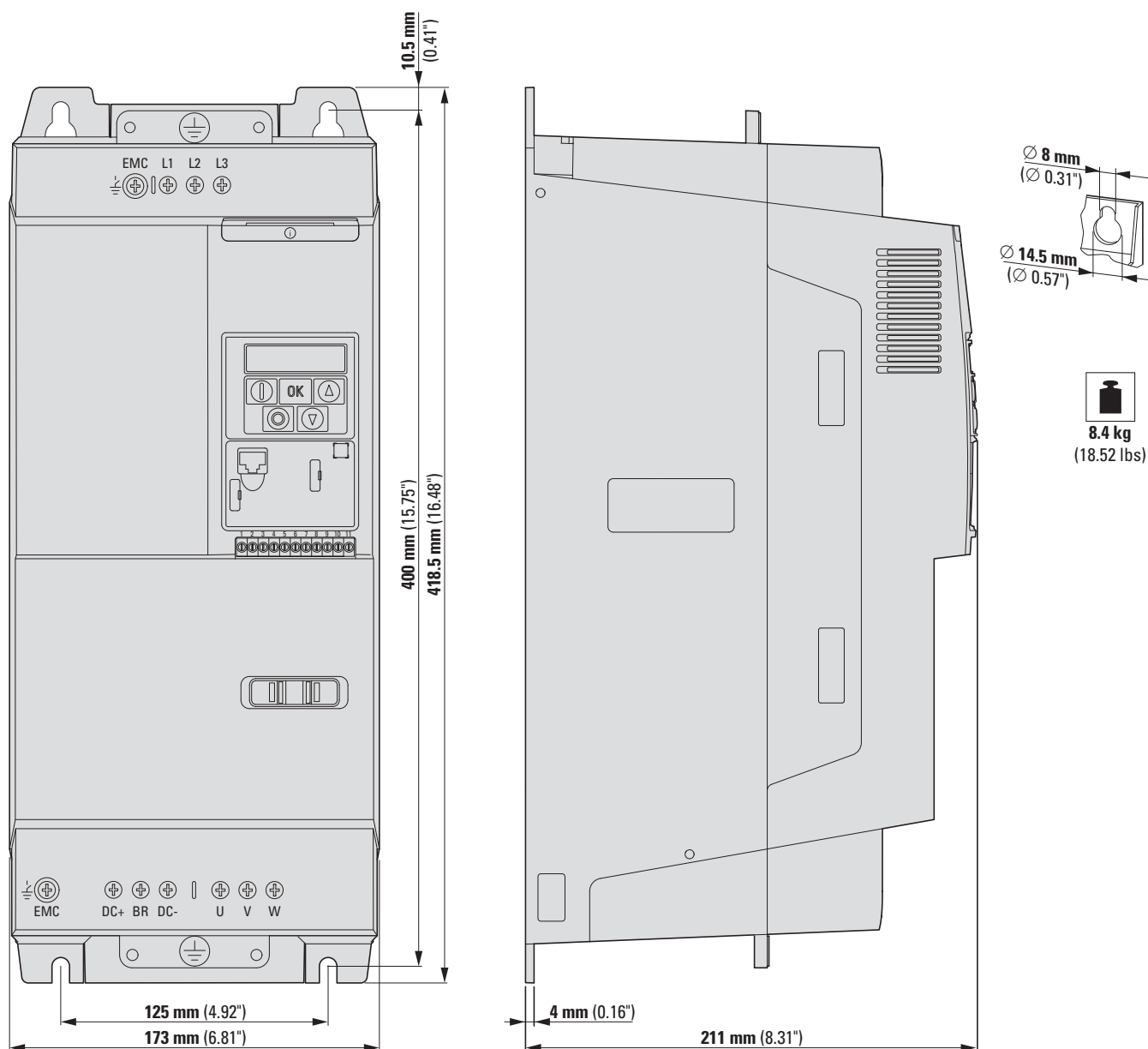
Figura 75: Dimensioni e peso DC1 di grandezza FS4 con grado di protezione IP20 (NEMA 0)
