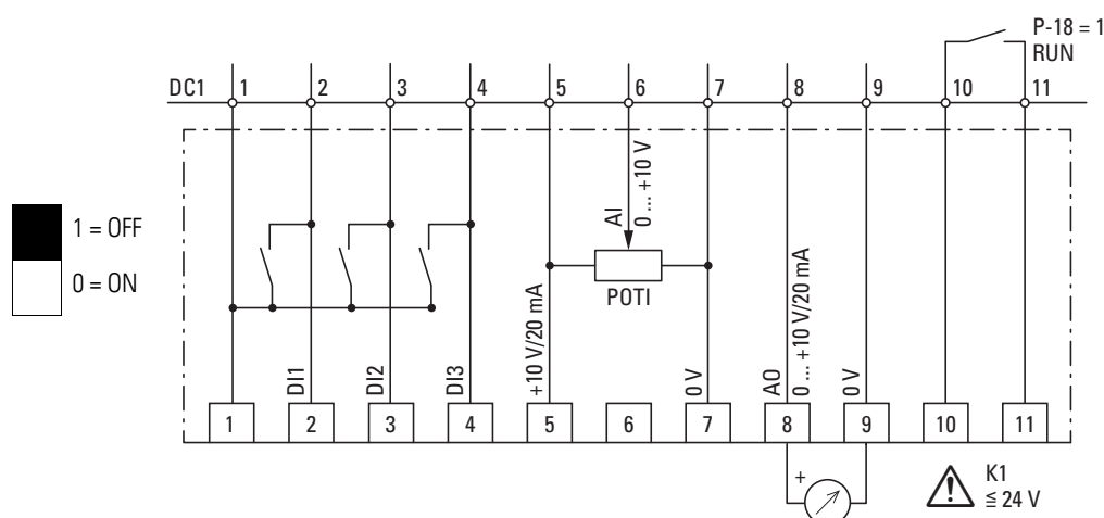
Figura 92: Schema a blocchi simulatore DXC-EXT-LOCSIM
