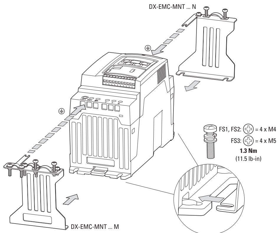
Figura 39: Portacavi EMC (esempio: grandezza FS2)
