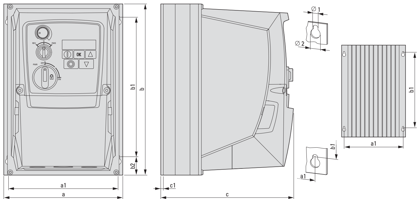
Figura 76: Dimensioni DC1 con grado di protezione IP66 (NEMA 4X)
