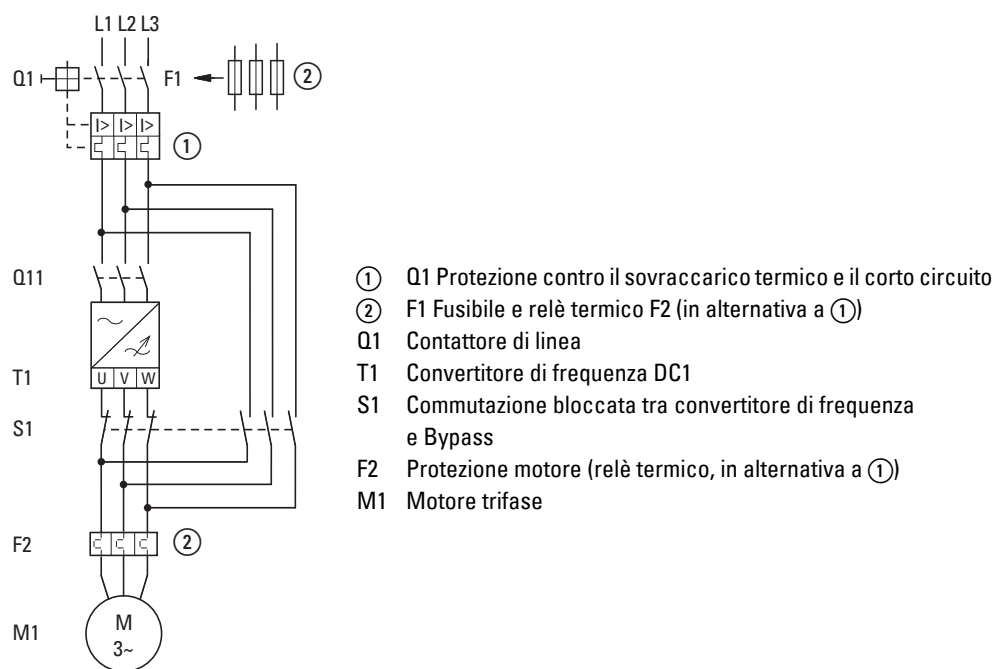
Figura 18: Comando motore a bypass (esempio)
