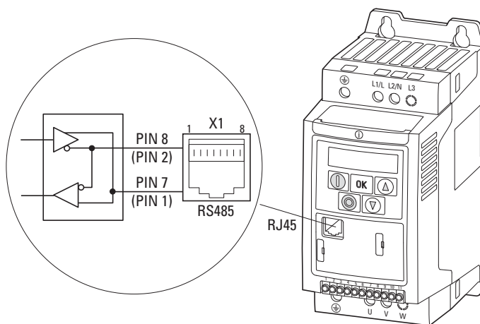
Figura 58: Interfaccia RJ45
