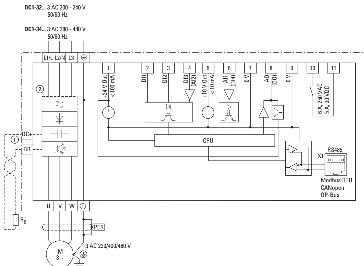
Figura 66: Schema a blocchi DC1-1D...Nx-A66...
