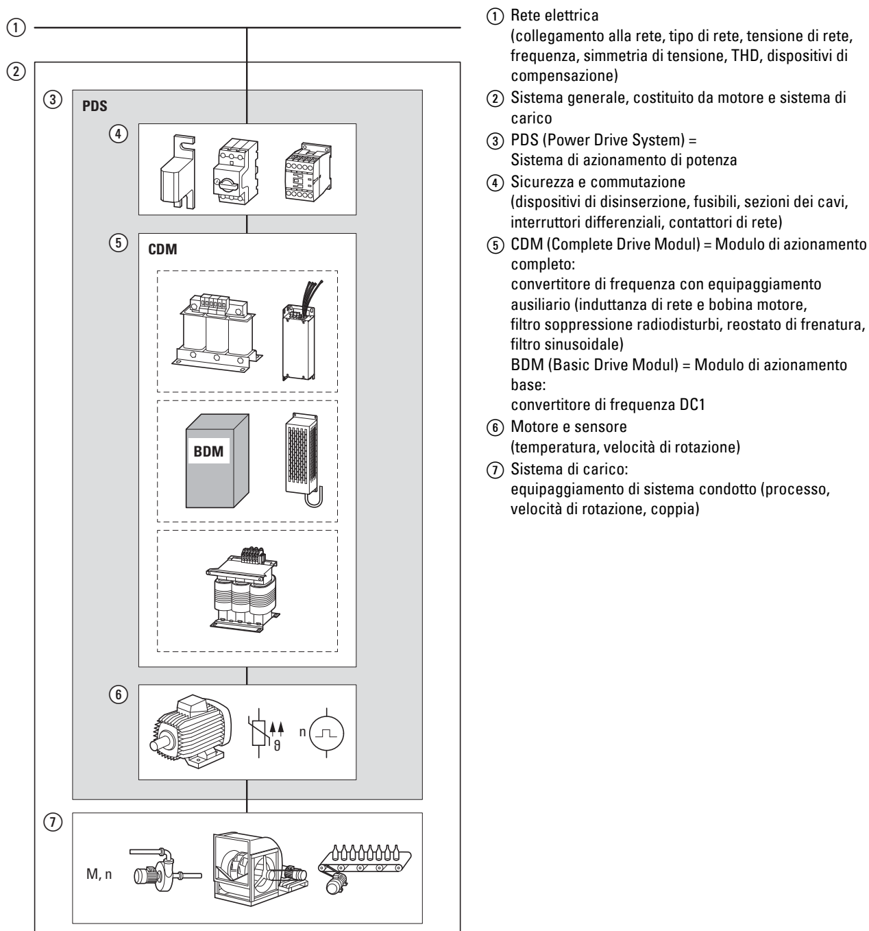
Figura 13: Esempio per un sistema di azionamento (sistema generale come impianto o parte di un impianto)
