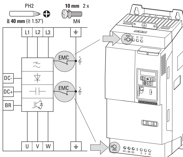
Figura 37: Due viti EMC per grandezza FS4
