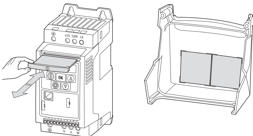
Figura 71: Schede ausiliare per il grado di protezione IP20 (a sinistra) e IP66 (a destra)
