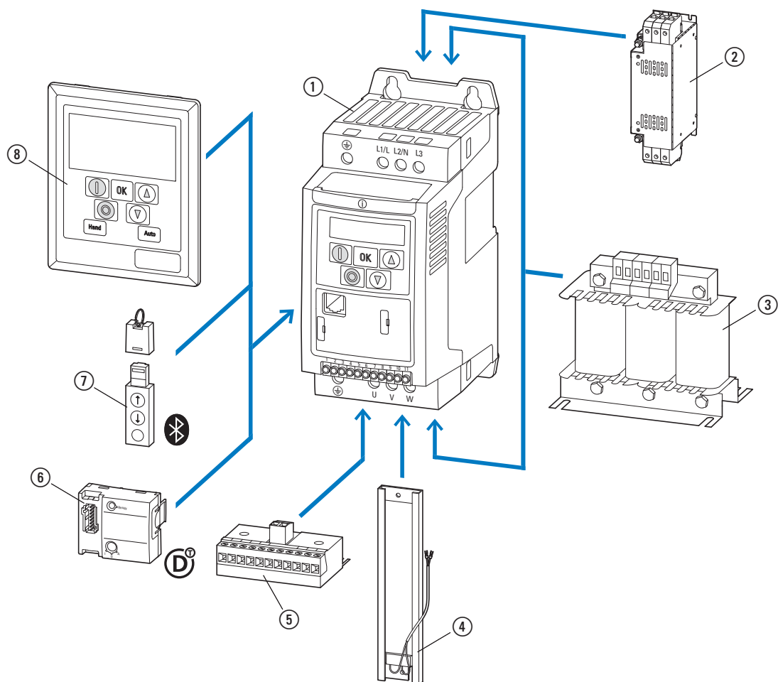
Figura 2: Composizione del sistema (Esempio: grandezza FS1, grado di protezione IP20)
