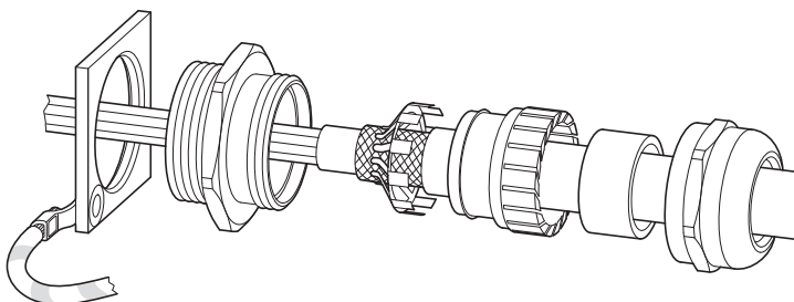
Figura 50: Esempio: struttura di principio del pressacavo EMC
