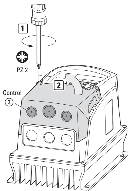
Figura 42: Rimozione della copertura inferiore della custodia
