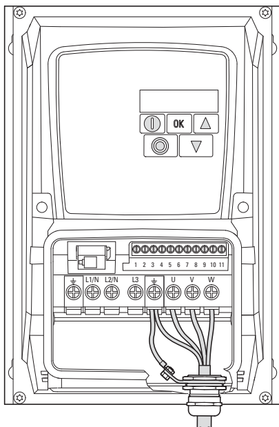
Figura 49: Messa a terra del pressacavo EMC
