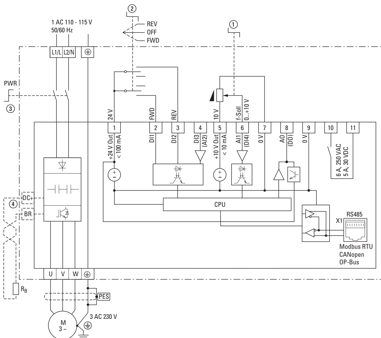
Figura 65: Schema a blocchi DC1-1D...Nx-A6S...
