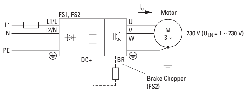
Figura 8: DC1-1D...
