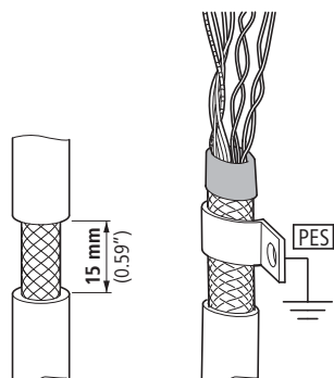
Figura 53: Allacciamento della schermatura (PES) su un solo lato in prossimità del convertitore di frequenza
