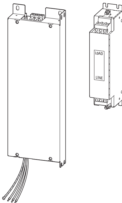
Figura 80: Filtri soppressione radiodisturbi esterni DX-EMC...-FS... (filtro installato nella base con cavo di collegamento preconfezionato) e DX-EMC...-L (filtro annesso)
