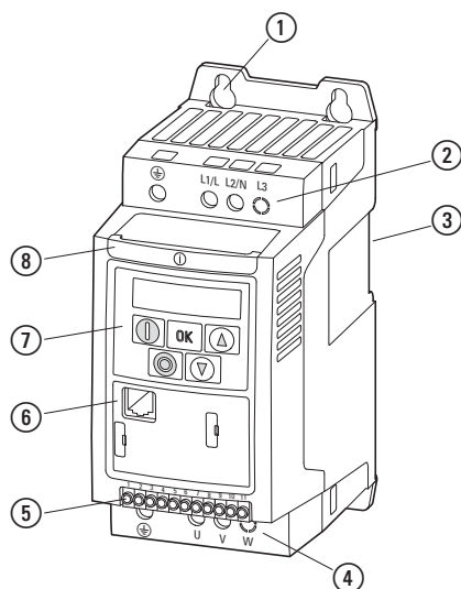
Figura 6: Denominazione su DC1 (FS1, IP20)
