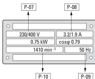
Figura 73: Targhetta dati macchina di un motore, P-08 = 1,9 A con 400 V
