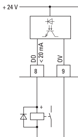
Figura 55: Esempio di cablaggio (relè di accoppiamento con diodo a ruota libera ETS4-VS3)
