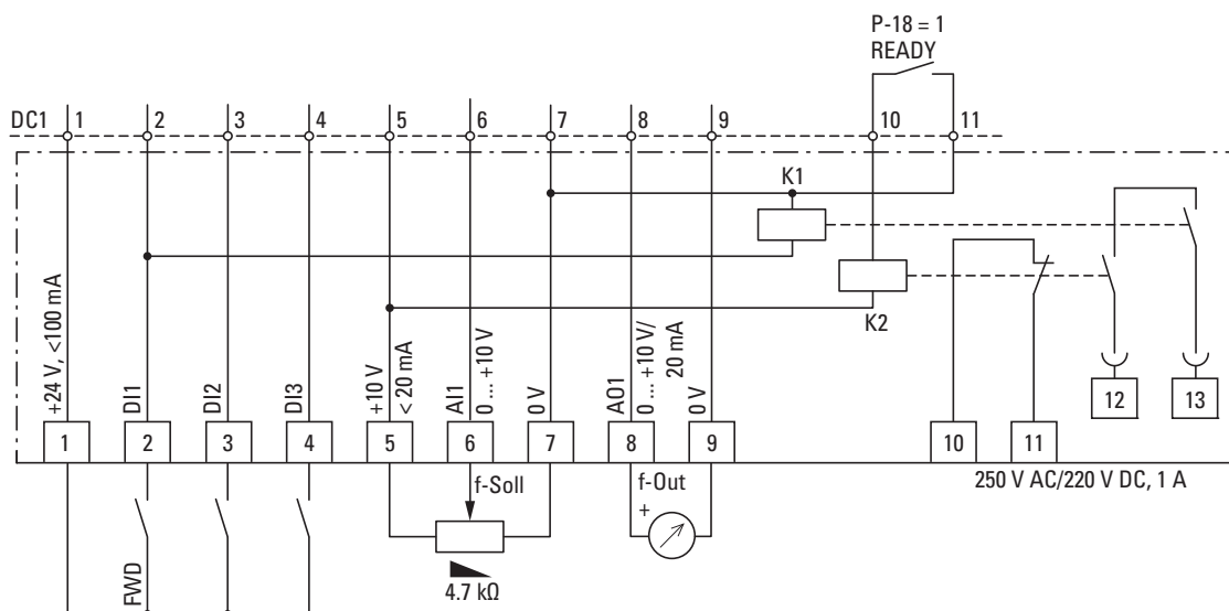
Figura 90: Schema a blocchi DXC-EXT-2RO1AO
