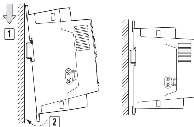
Figura 29: Fissaggio su una guida di montaggio
