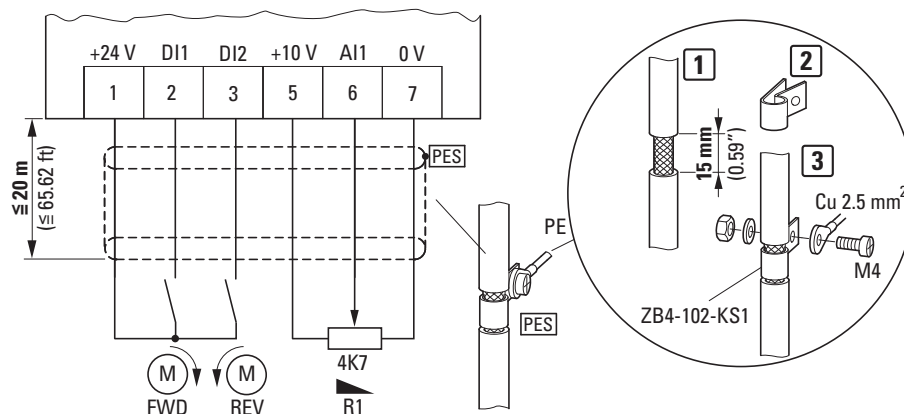
Figura 52: Semplice esempio di collegamento
