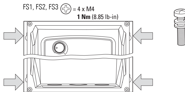
Figura 32: Aperture per le viti di fissaggio
