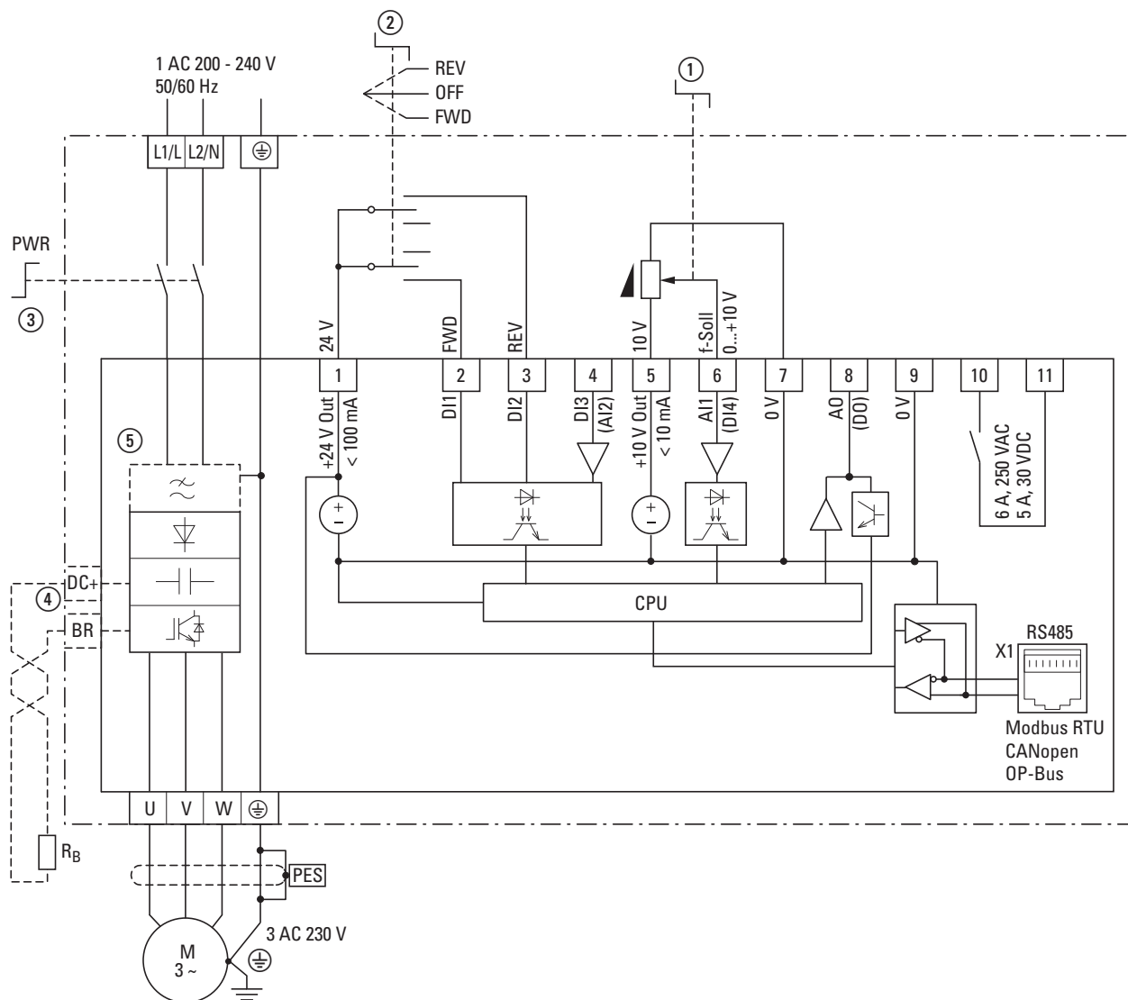
Figura 67: Schema a blocchi DC1-12...-A6S...
