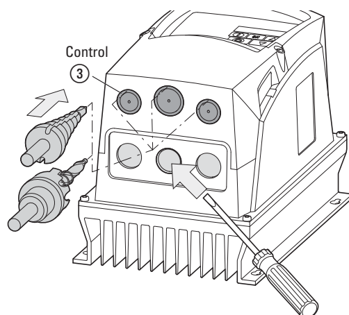
Figura 47: Sfondare le aperture (esempio)
