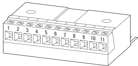
Figura 87: DXC-EXT-2RO
