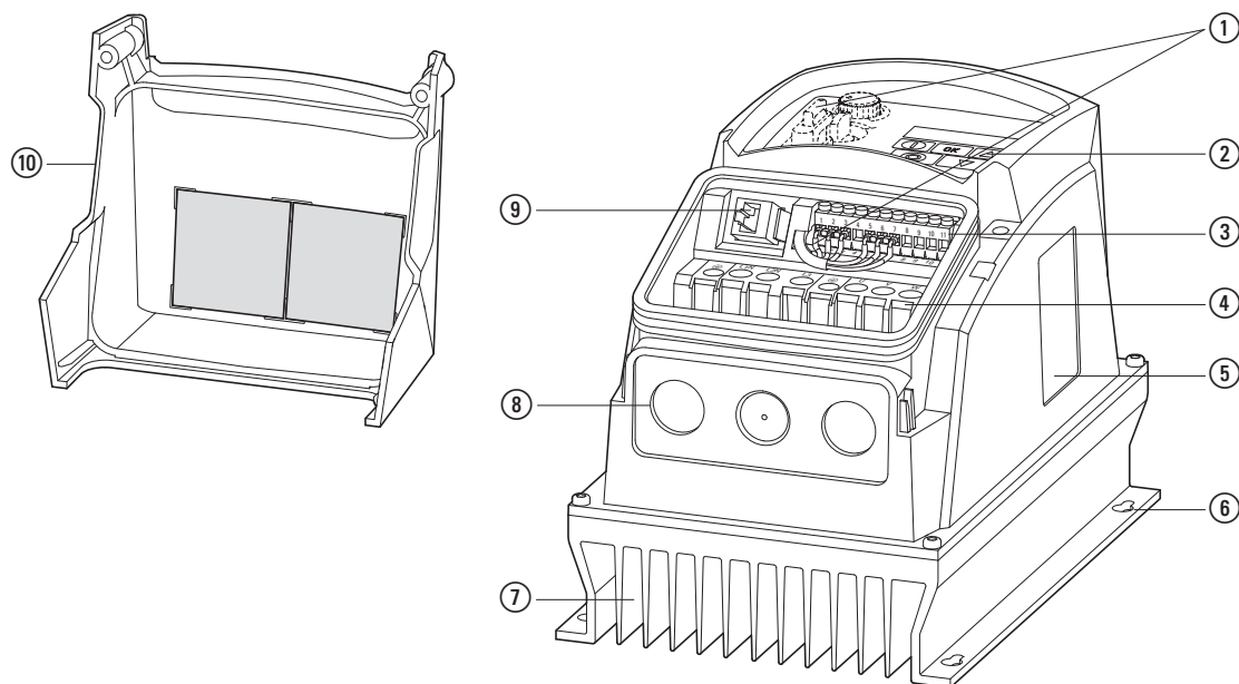
Figura 7: Denominazione (IP66)
