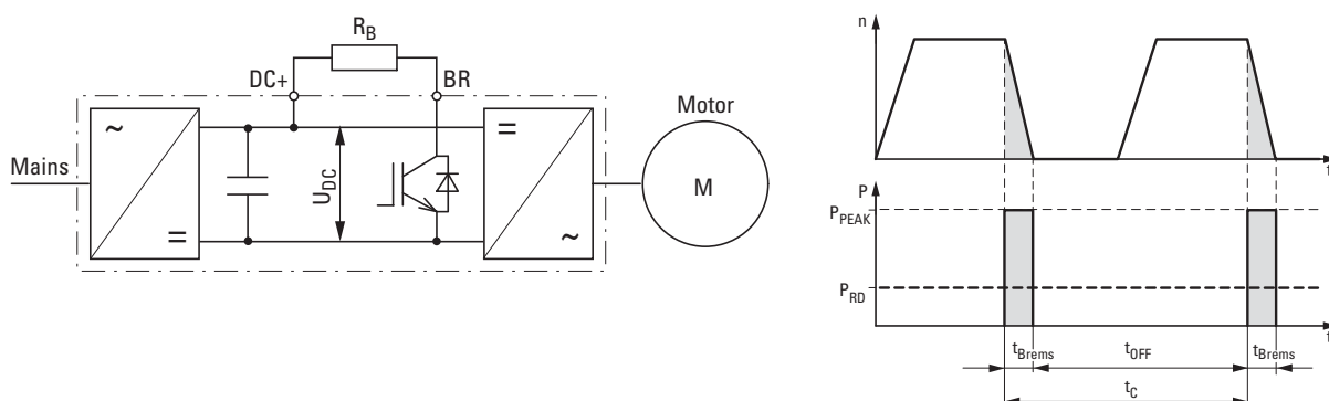
Figura 16: Ciclo di frenatura, arresto motore rapido con reostato di frenatura esterno
