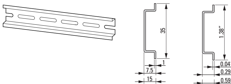
Figura 28: Guida di montaggio a norma IEC/EN 60715
