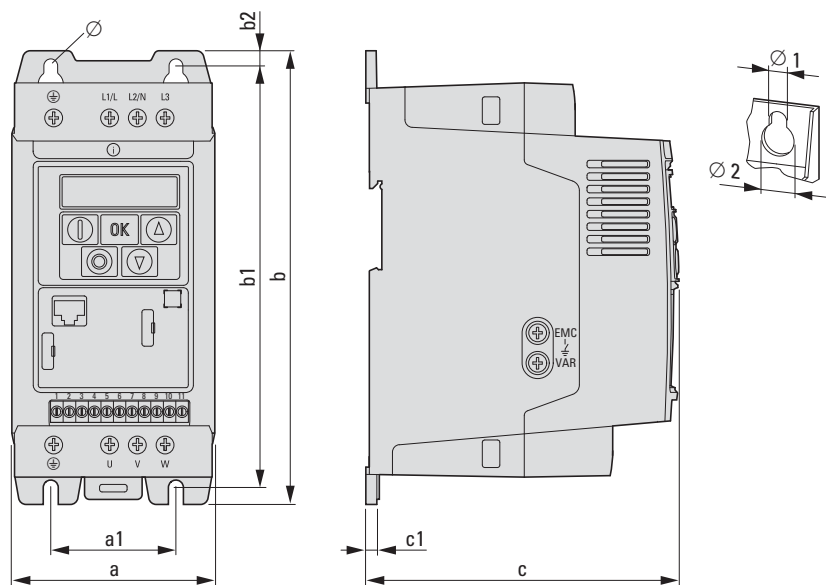
Figura 74: Dimensioni DC1 con grado di protezione IP20 (NEMA 0)
