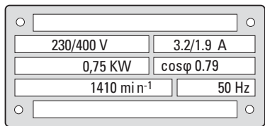
Figura 20: Esempio di targa dati (targhetta dati macchina) di un motore asincrono a corrente alternata trifase
