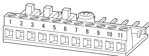
Figura 91: DXC-EXT-LOCSIM
