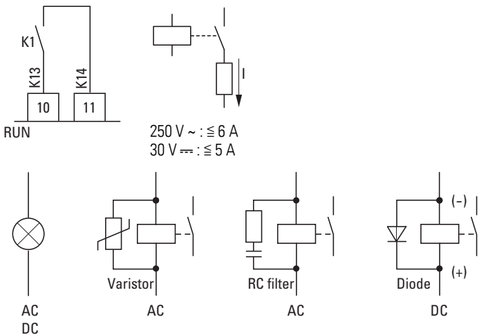
Figura 57: Esempi di cablaggio con circuito di protezione
