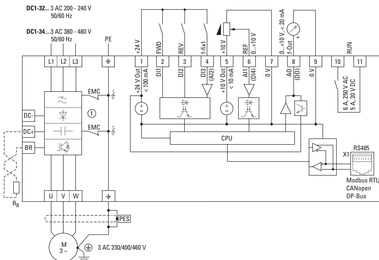
Figura 64: Schema a blocchi DC1-32... e DC1-34... nella grandezza FS4
