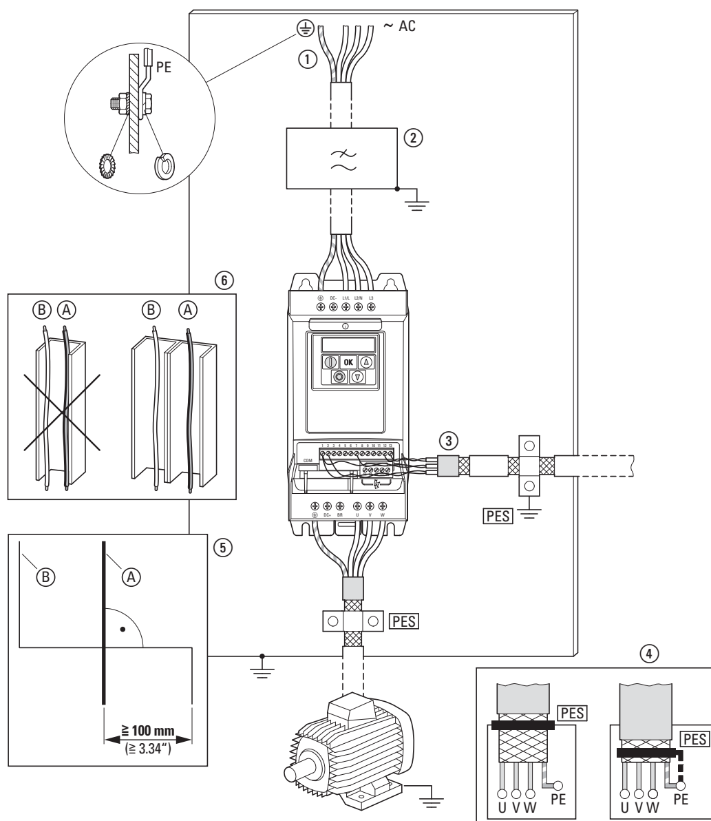
Figura 40: Installazione a norma EMC
