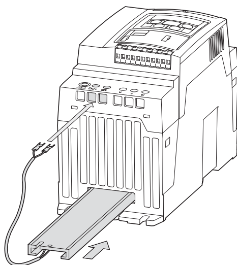
Figura 15: Convertitore di frequenza DC1 di grandezza FS2 con reostato di frenatura DX-BR3-100
