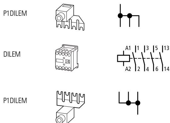
Figura 77: Contattore di linea per collegamento monofase (DC1-12...)
