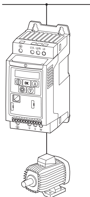
Figura 41: Collegamento nello stadio di potenza (principio)
