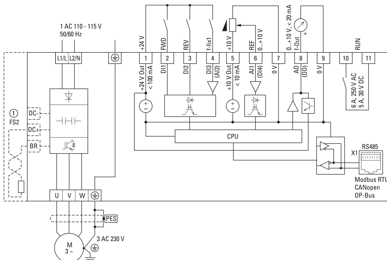
Figura 61: Schema a blocchi DC1-1D...Nx...
