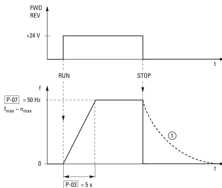
Figura 69: Comando di avvio/arresto alla massima tensione di riferimento, rampa di accelerazione 5 s
