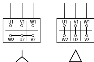
Figura 21: Tipi di circuito: collegamento a stella (a sinistra), collegamento a triangolo (a destra)
