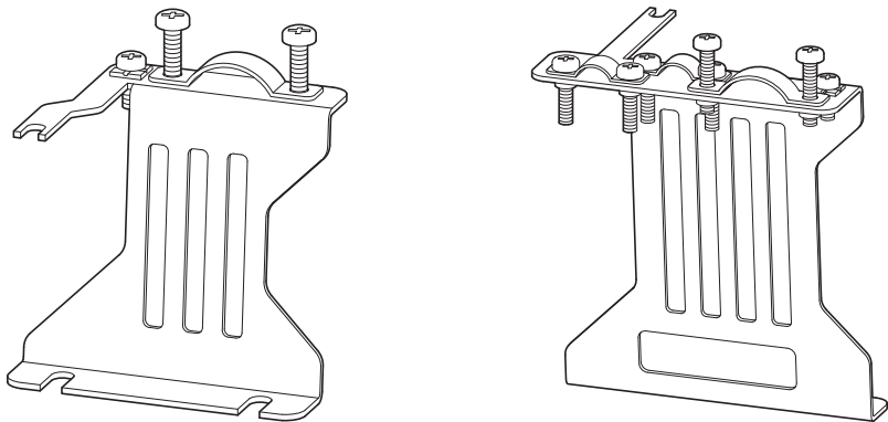
Figura 38: Portacavi DX-EMC-MNT-...N (a sinistra), rete e DX-EMC-MNT-...M (a destra), motore
