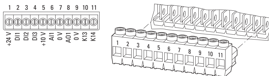
Figura 51: Disposizione e denominazione da parte del costruttore dei morsetti di comando
