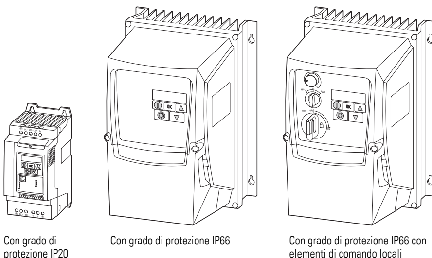
Figura 1: Esecuzione e varianti di custodia
