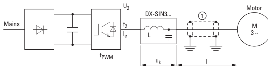
Figura 83: Lunghezze massime consentite dei cavi motore
