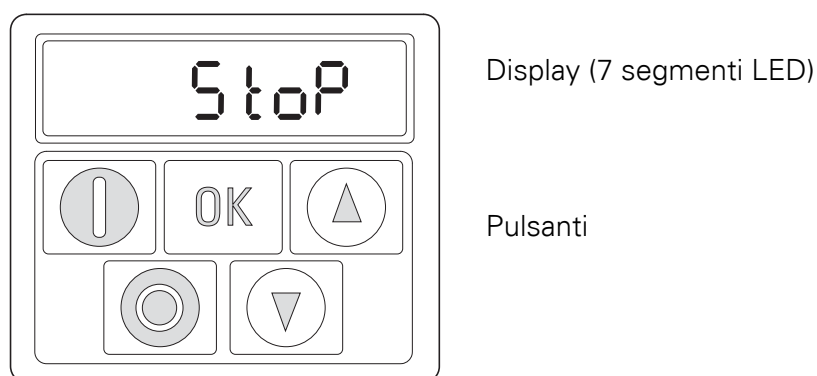
Figura 70: Vista dell'organo di comando (esempio DC1-...-A20...)
