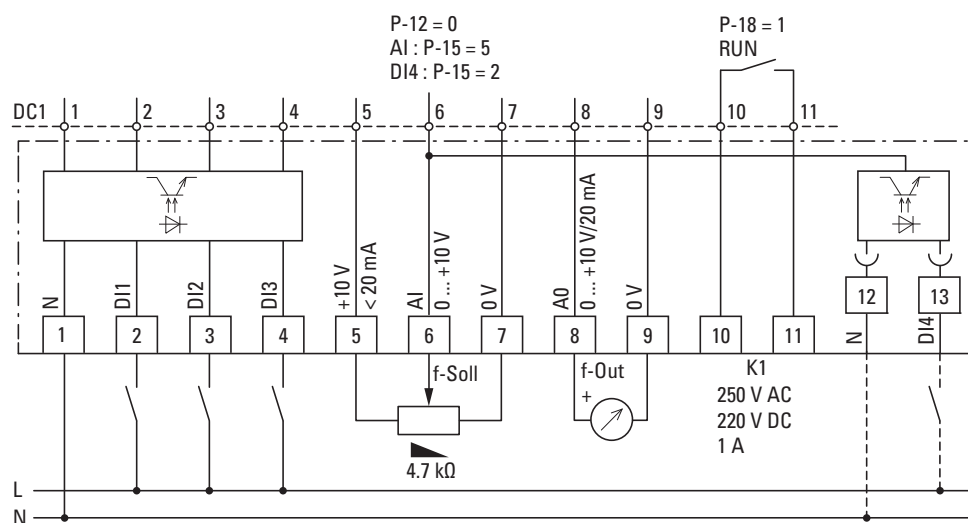
Figura 86: Schema a blocchi DXC-EXT-IO110 e DXC-EXT-IO230
