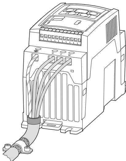
Figura 44: Collegamento sul lato motore
