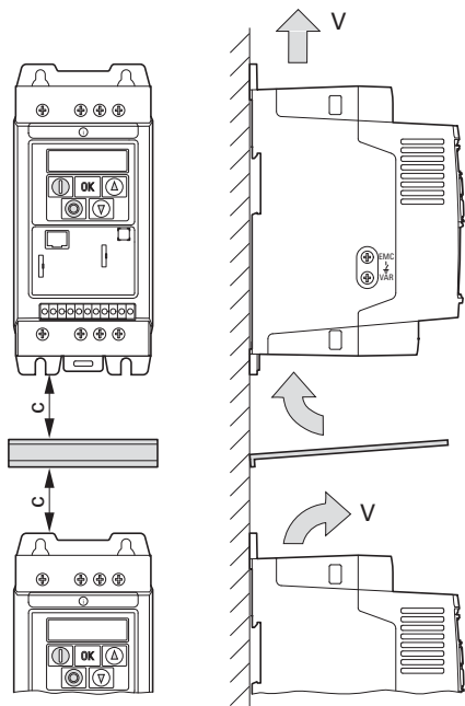
Figura 25: Deflettore in caso di una massiccia circolazione ad opera del ventilatore
