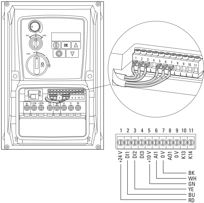
Figura 59: DC1-...A6S... (collegamento in fabbrica) Nello stato alla consegna i morsetti di comando sono collegati come segue:
