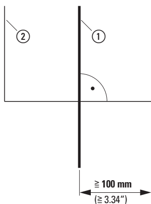
Figura 34: passaggio cavi
