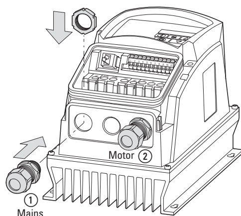
Figura 48: Montaggio dei pressacavi
