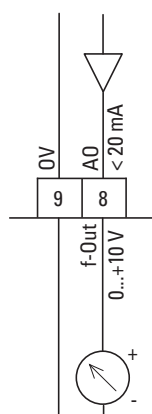
Figura 56: Uscita analogica (AO) (esempio di cablaggio)
