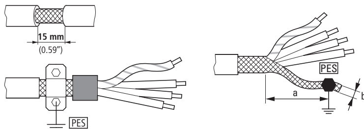
Figura 45: Cavo di collegamento schermato nel circuito motore
