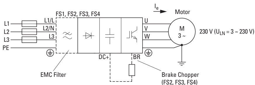
Figura 10: DC1-32...
