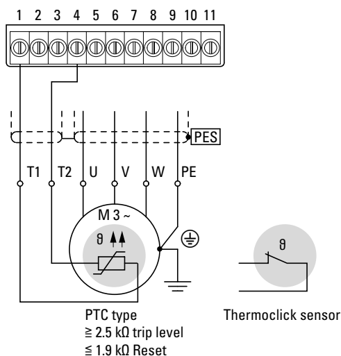
Figura 60: Collegamento del termistore
