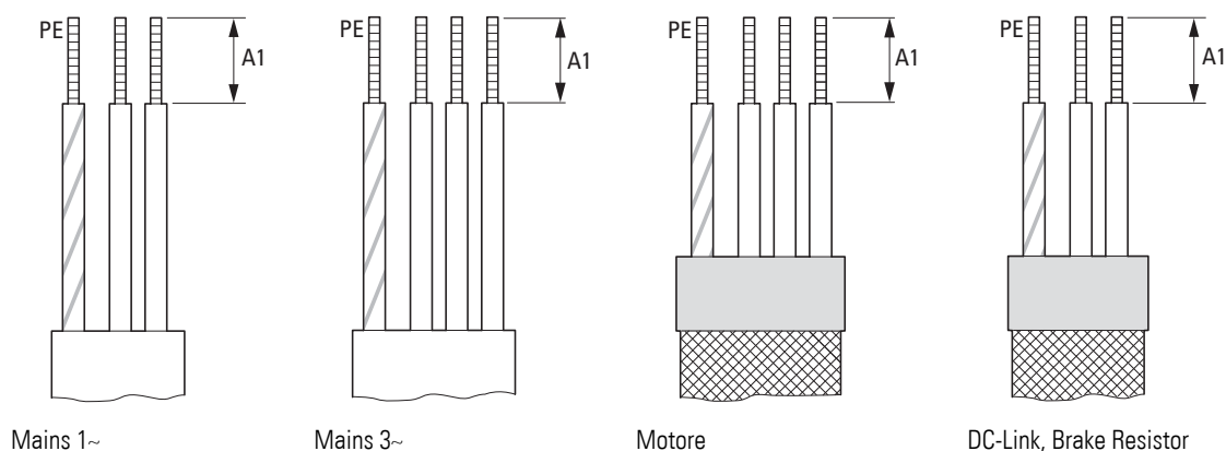
Figura 43: Lunghezze di spelatura nello stadio di potenza
