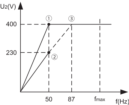
Figura 14. Curva caratteristica V/Hz
