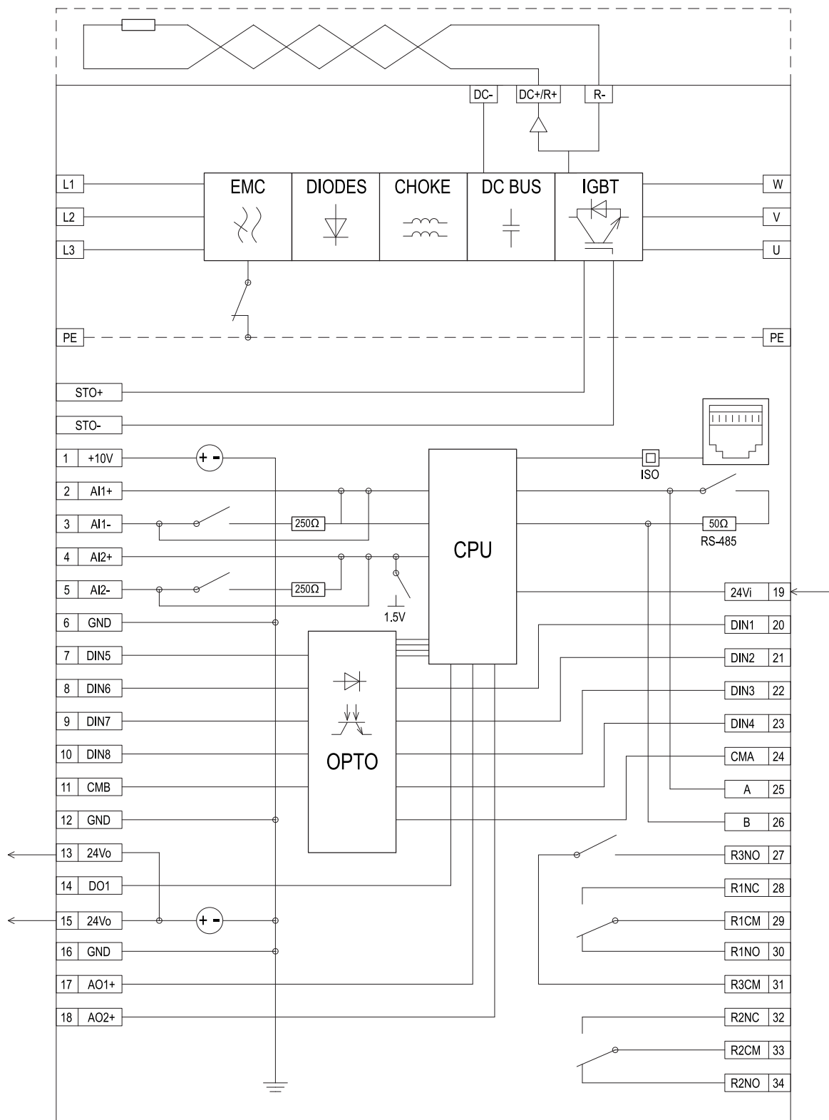
Figura 21. Schema base di cablaggio comando interno
