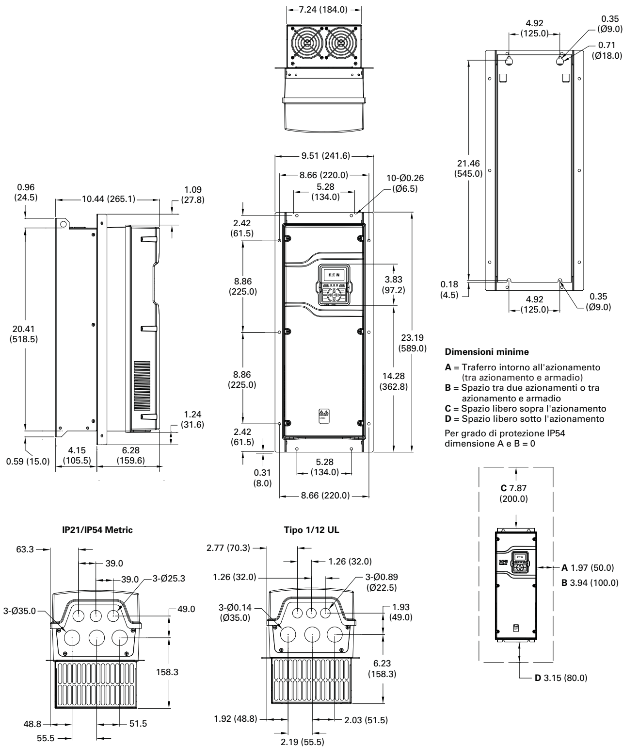
Figura 37. FR3 Disegno quotato montaggio flangia
