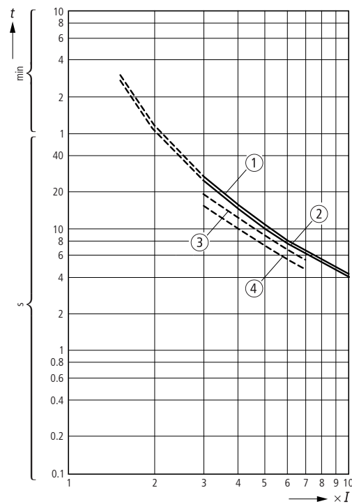
Abbildung/Figure 16: ZE-0,6/XTOMP60AC1
