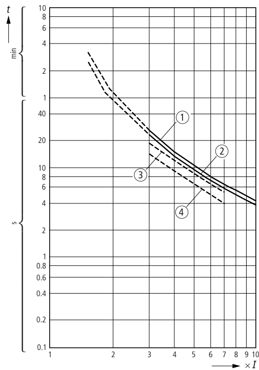
Abbildung/Figure 17: ZE-1,0/XTOM001AC1
