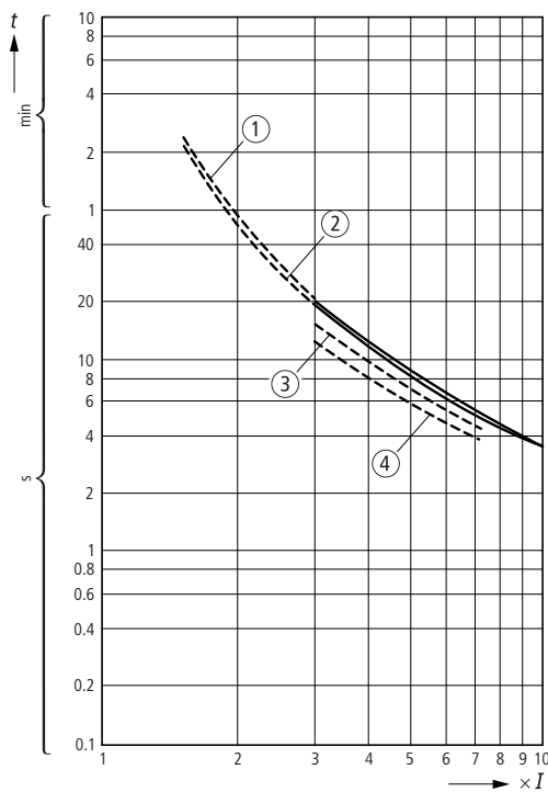
Abbildung/Figure 13: ZE-0,16/XTOMP16AC1
