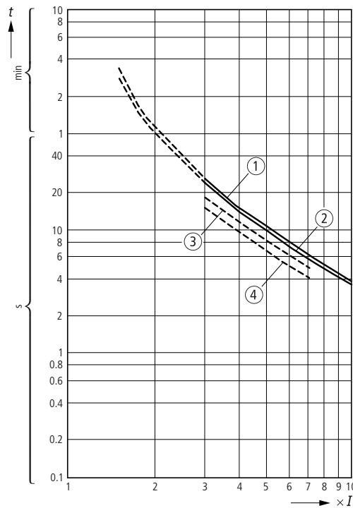
Abbildung/Figure 21: ZE-6/XTOM006AC1
