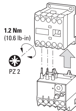
Abbildung 7: Montage DIL(E)EM/XTMC und ZE/XTOM
