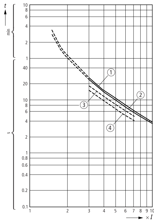
Abbildung/Figure 22: ZE-9/XTOM009AC1
