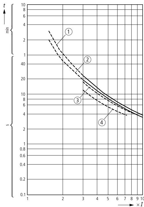
Abbildung/Figure 15: ZE-0,4/XTOMP40AC1
