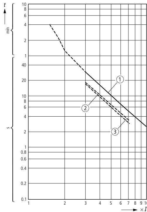
Abbildung/Figure 23: ZE-12/XTOM012AC1
