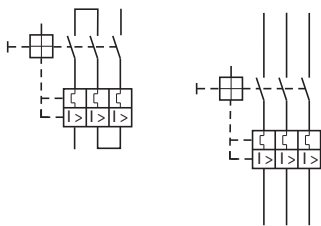
Abbildung 8: Hauptstromverdrahtung
